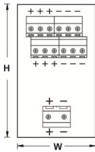
Dimensions
